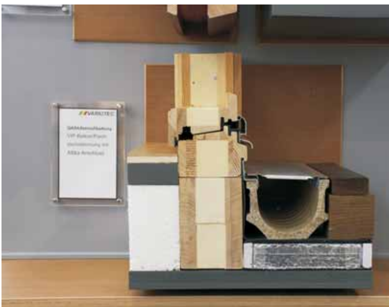
QASAflatroof/balkony: VIP-Balkon/Flachdachdämmung mit Attika-Anschluss
