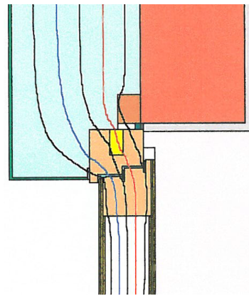
Schwelle Eingangstür
