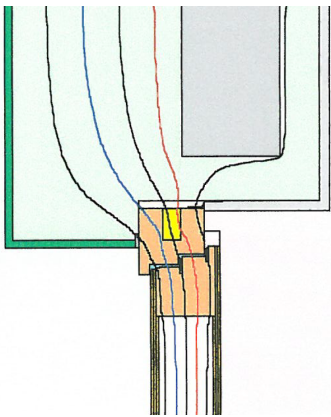
Holzleichtbau (öffnbar)
